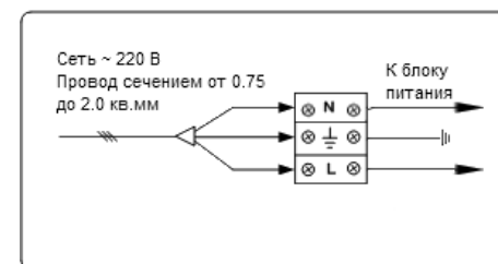
Рис. 1. Схема подключения к сети
